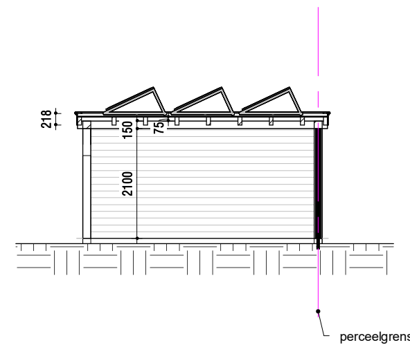
Doorsnede
