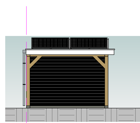
Linkergevel
